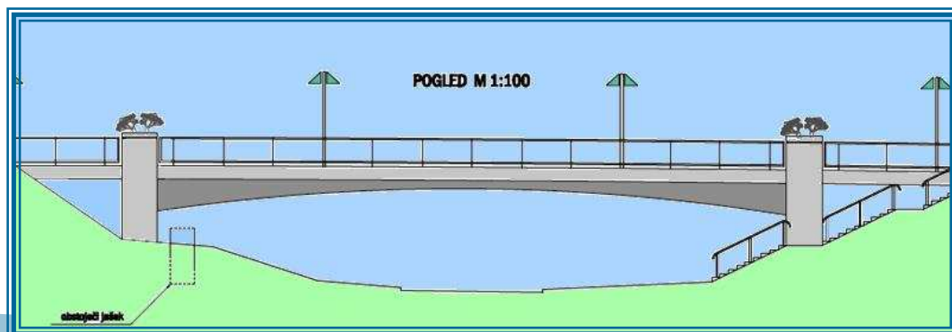
Načrtovani novi nadvoz
